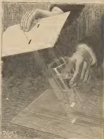
Experimento acerca de la refracción de la luz por medio de un prisma obtenido con un vaso de agua.
